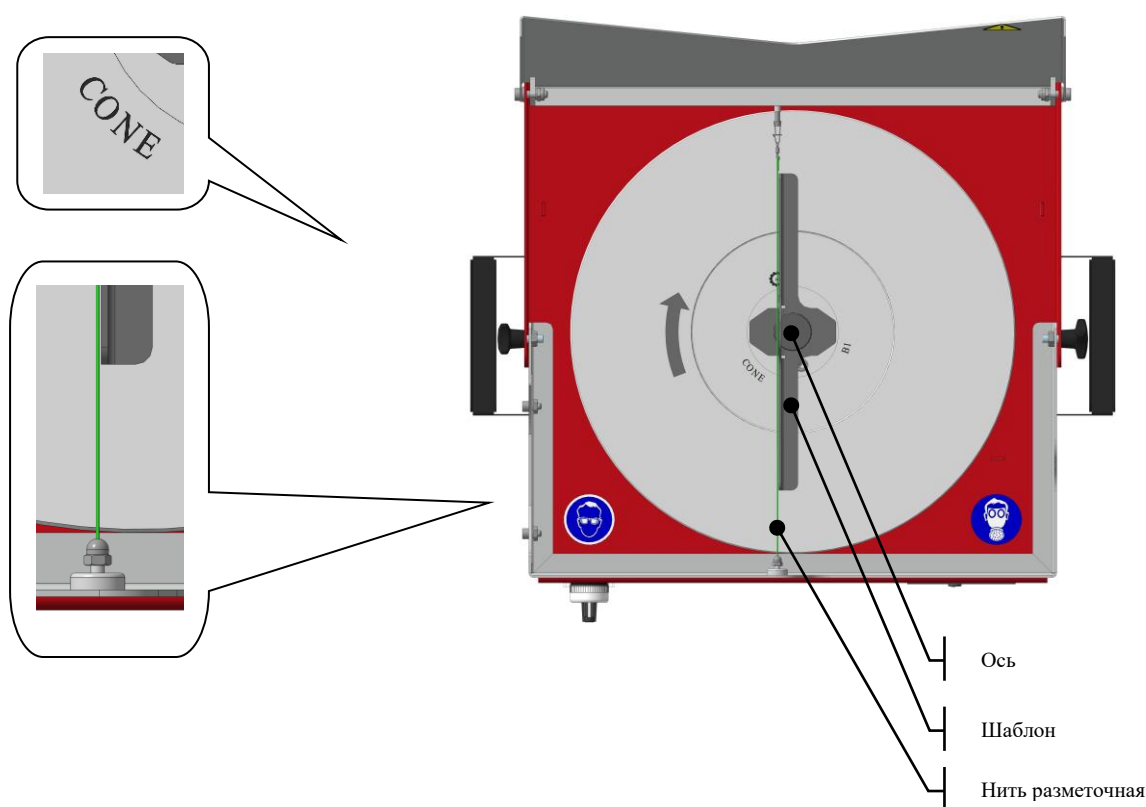
Рис.3 Настройка положения ножа при заточке
