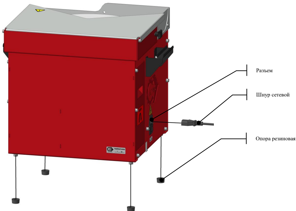
Рис.1 Сборка станка ADEMS Front Plate Inverter
