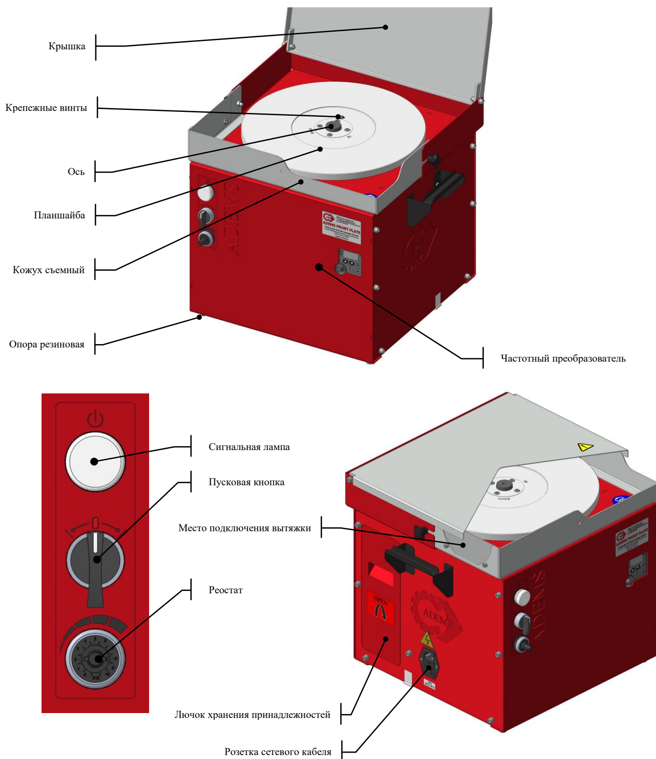
Рис. 2 Бытовой заточной станок ADEMS Front Plate Inverter
