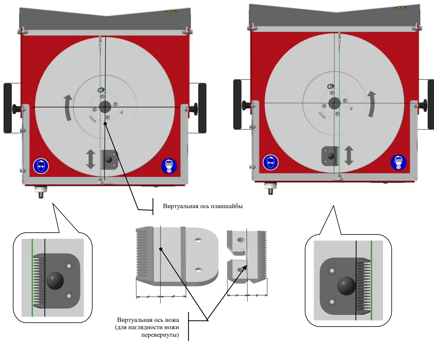
Рис.4 Положение ножа на планшайбе
